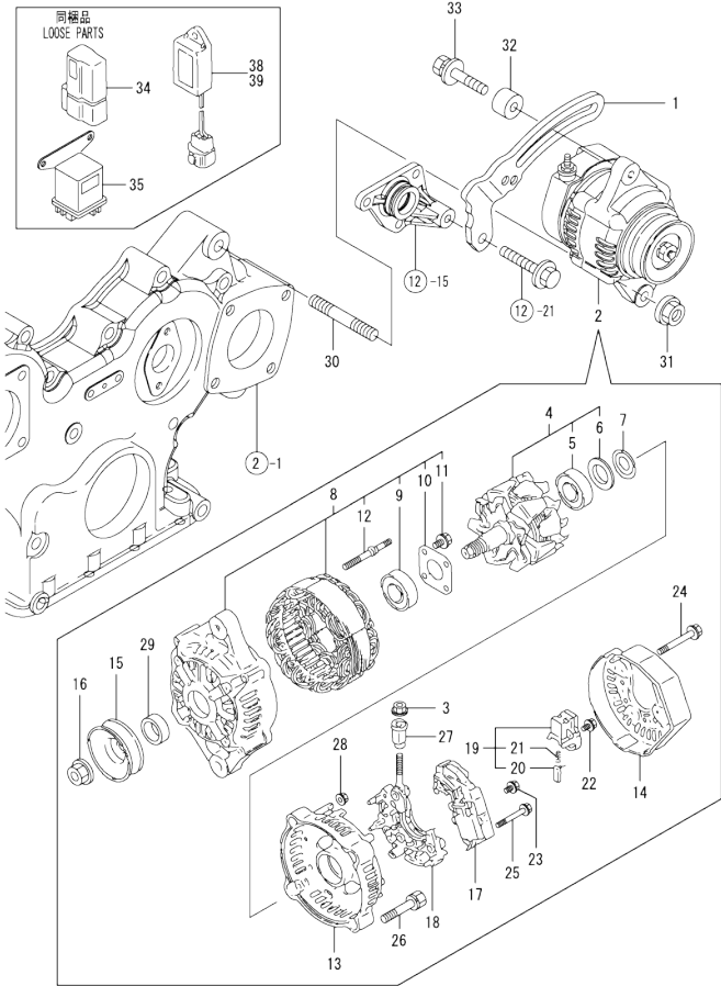
Fig.18. GENERATOR
